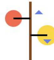
Cinética
